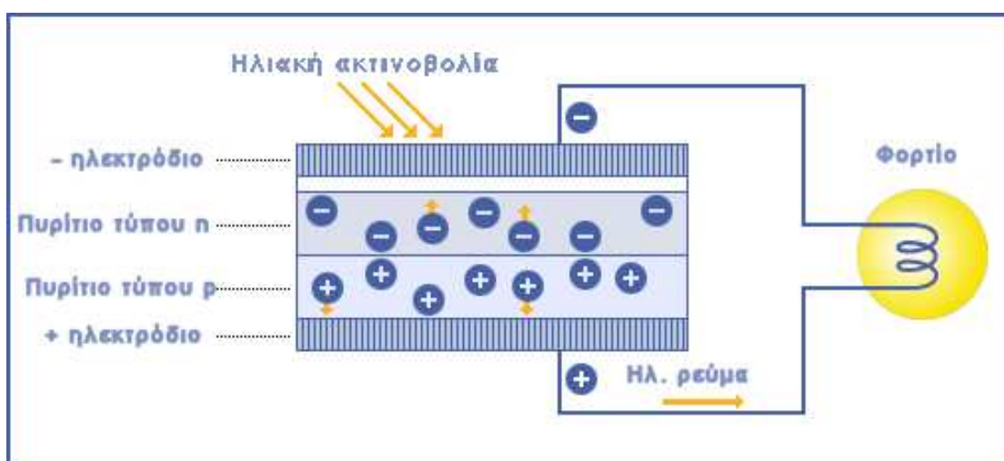
Αρχή λειτουργίας φωτοβολταϊκού φαινομένου
