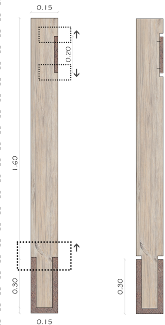
Εικόνα 57_Δομή γραμμικών στοιχείων αστικού εξοπλισμού και σύνθεση των επιλεγμένων υλικών, Πηγή: Ίδια επεξεργασία
