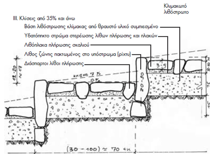
Εικόνα 3_Διάταξη λίθων σε διαφορετικούς τύπους πλακόστρωσης μονοπατιών, Πηγή: Παγκρατίου Ελ., Μιχαήλ Γ., Πουλογιάννη Ν., 2009, «Εγχειρίδιο ξερολιθικών κατασκευών: Λιθοστρώσεις»
