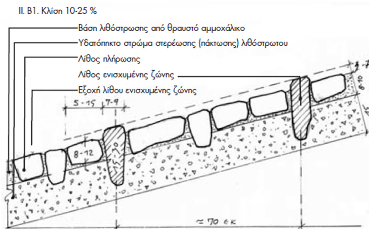
Εικόνα 3_Διάταξη λίθων σε διαφορετικούς τύπους πλακόστρωσης μονοπατιών, Πηγή: Παγκρατίου Ελ., Μιχαήλ Γ., Πουλογιάννη Ν., 2009, «Εγχειρίδιο ξερολιθικών κατασκευών: Λιθοστρώσεις»
