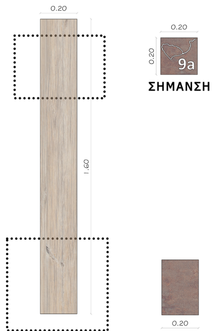
Εικόνα 57_Δομή γραμμικών στοιχείων αστικού εξοπλισμού και σύνθεση των επιλεγμένων υλικών, Πηγή: Ίδια επεξεργασία
