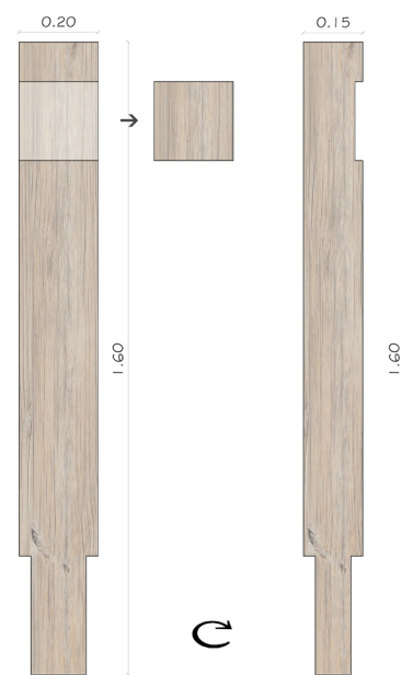
Εικόνα 57_Δομή γραμμικών στοιχείων αστικού εξοπλισμού και σύνθεση των επιλεγμένων υλικών, Πηγή: Ίδια επεξεργασία
