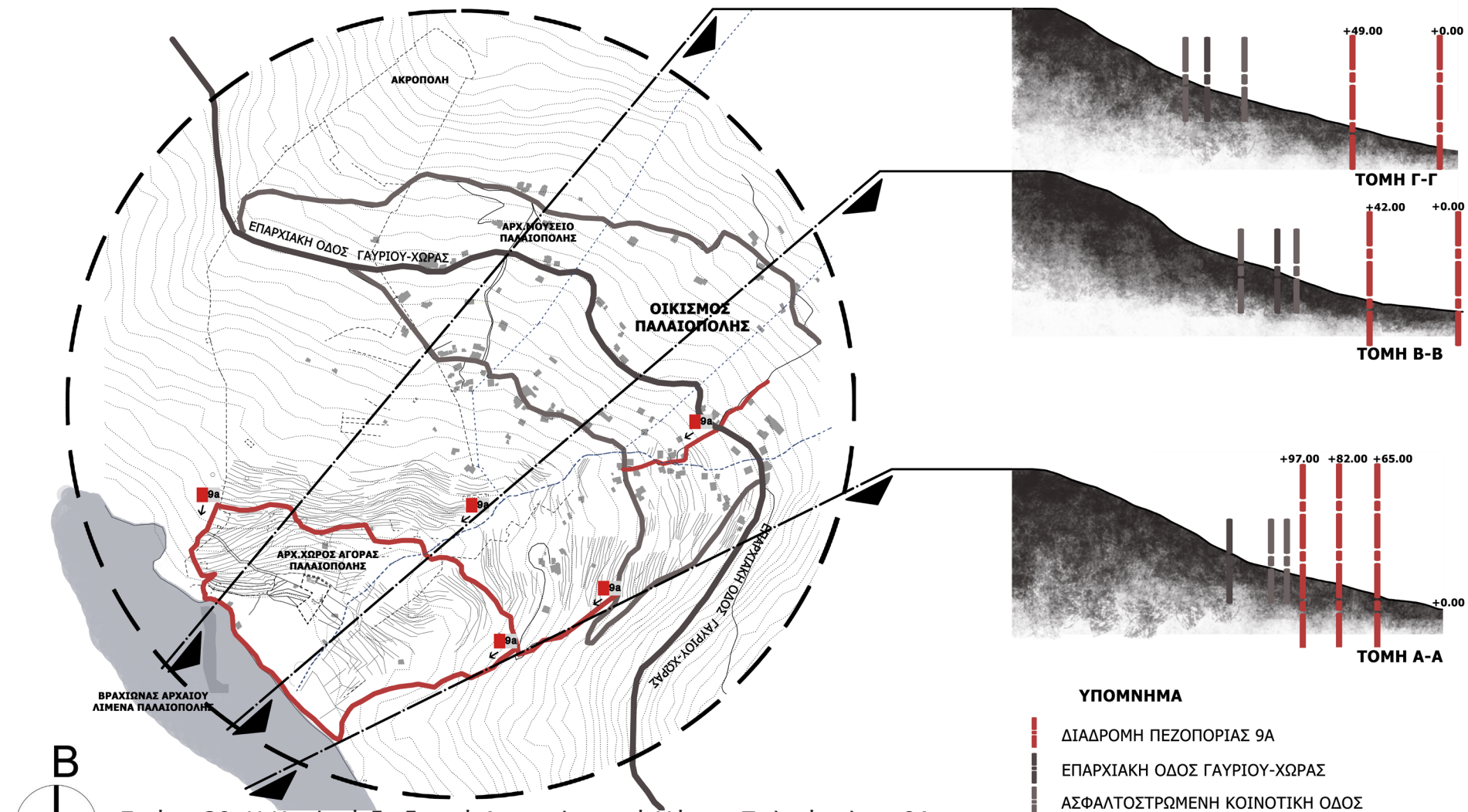
Εικόνα 30_Η Κυκλική διαδρομή Αρχαιολογικού Χώρου Παλαιόπολης, 9Α, Τομές αναγλύφου της περιοχής, Πηγή: Ίδια επεξεργασία
