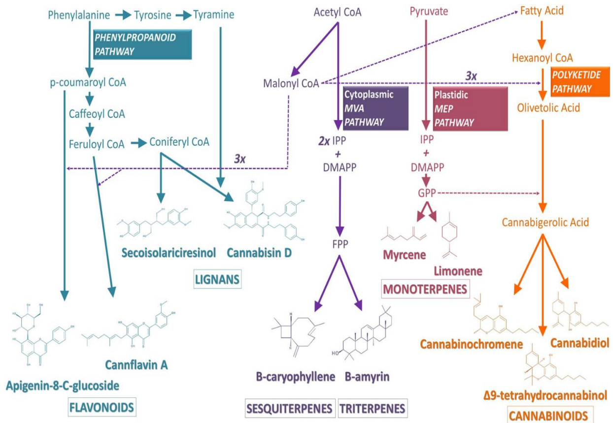
Εικόνα 12. Σχηματική απεικόνιση του βιοσυνθετικού μονοπατιού που οδηγεί σε δευτερογενείς μεταβολίτες της κάνναβης ( Cannabis sativa L.)(Benvenuto, Misra et al. 2016).
