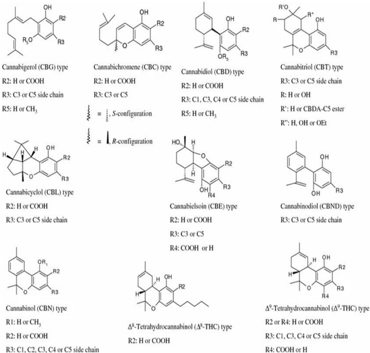
Εικόνα 10. Οι δέκα βασικοί δομικοί τύποι κανναβινοειδών στα οποία ταξινομούνται τα κανναβινοειδή που έχουν ως τώρα απομονωθεί (Flores-Sanchez and Verpoorte 2008).
